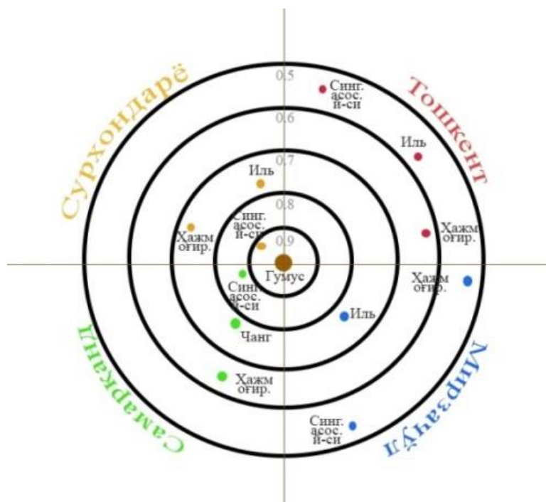
7-расм. Турли регионлар воҳа тупроқларидаги гумус ва бошқа хусусиятларнинг ўзаро таъсири куёш корреляцион диаграммаси (К.Пирсон услуби бўйича)
