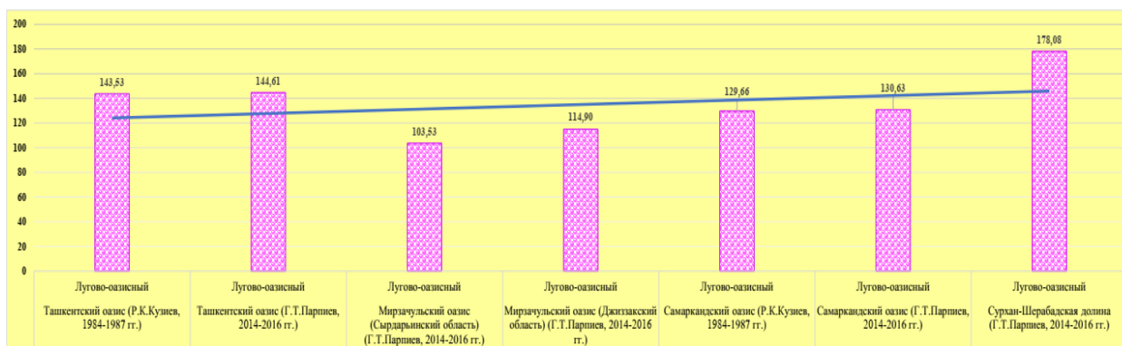
Рисунок 6. Запасы гумуса в 1 метровом слое лугово-оазисных почв, т/га.
