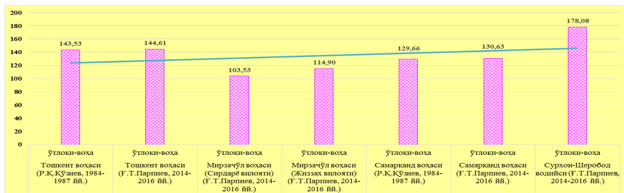
6-расм. Ўтлоқи-воҳа тупроқларнинг бир метрлик қатламидаги гумуснинг заҳираси, т/га.
