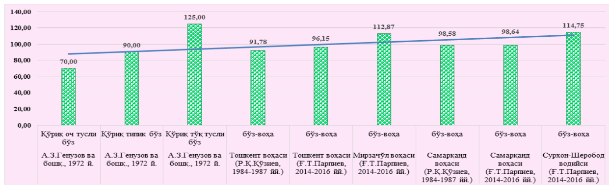
4-расм. Бўз-воҳа тупроқларнинг бир метрлик қатламидаги гумуснинг заҳираси, т/га.
