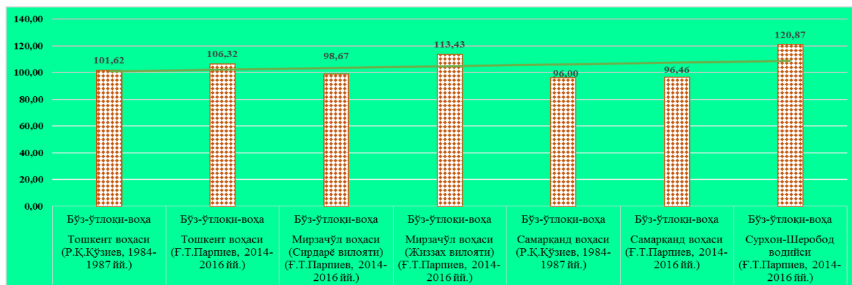
5-расм. Бўз-ўтлоқи-воҳа тупроқларнинг бир метрлик қатламидаги гумуснинг заҳираси, т/га.
