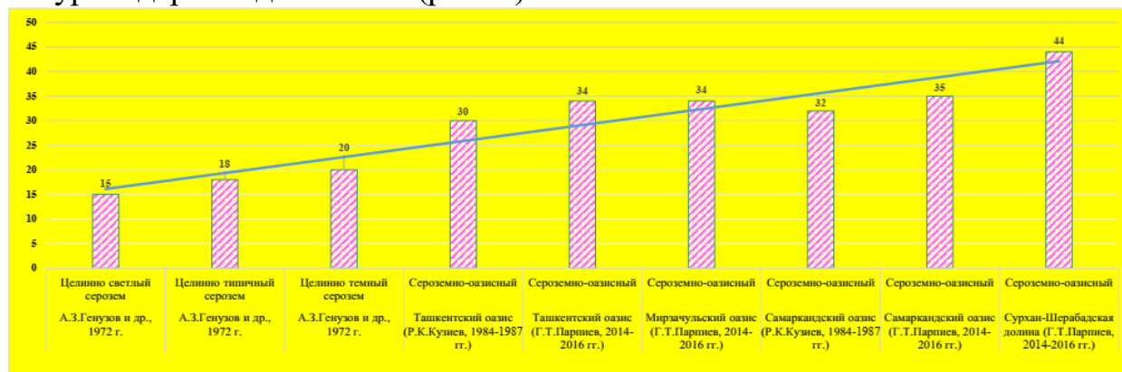
Рисунок 1. Мощность аккумулятивного гумусного (А) горизонта сероземно-оазисных почв
